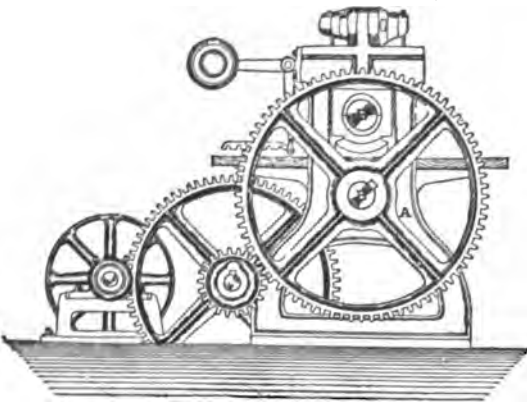
FIG. 10.—Plate Calender.
