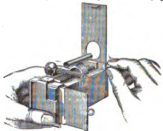
FIG. 9.—Marion & Co.'s Camera.
